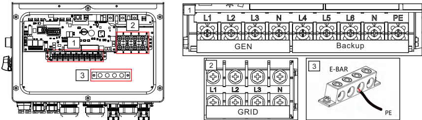
图 3.17 交流输出端子
